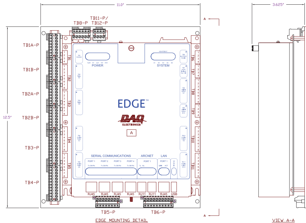
EDGE MOUNTING DETAIL
